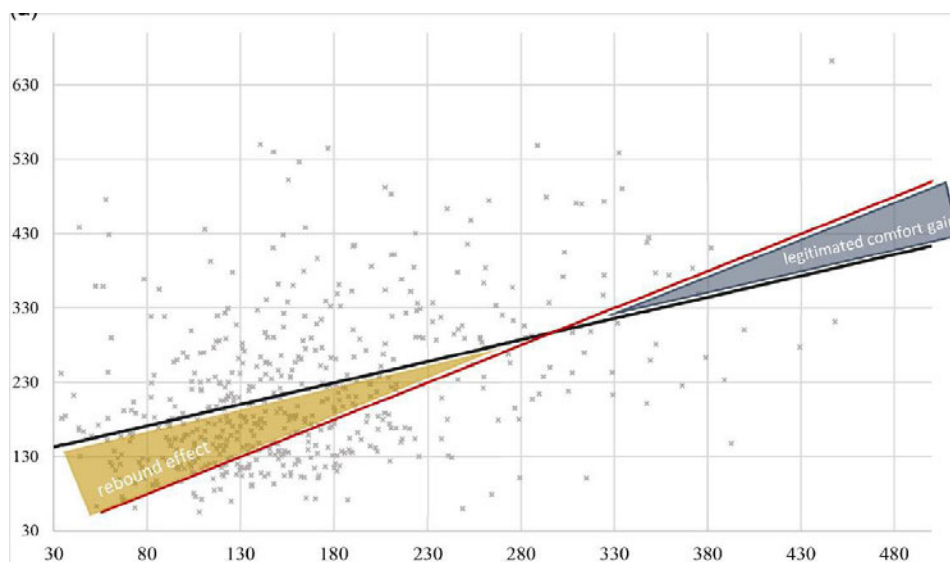
Graphique 1 : Relation entre les consommations d'énergie réelles et théoriques
