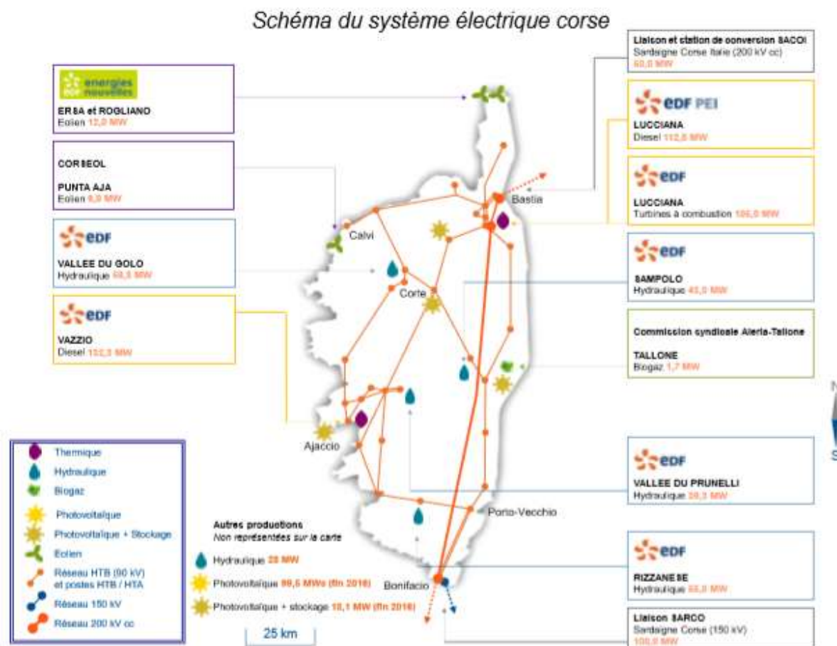
Graphique 5 : Le réseau électrique de Corse
